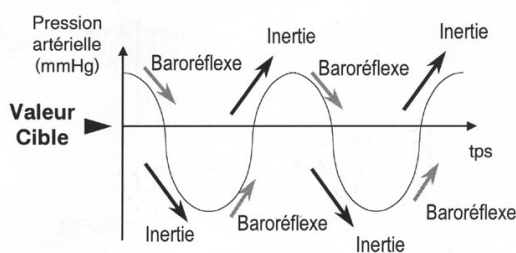
Figure 1 : Résonance du Baroréflexe : oscillation de la PA autour de la valeur cible, engendrée par le retard entre l'afférence et l'efférence de l'arc réflexe
